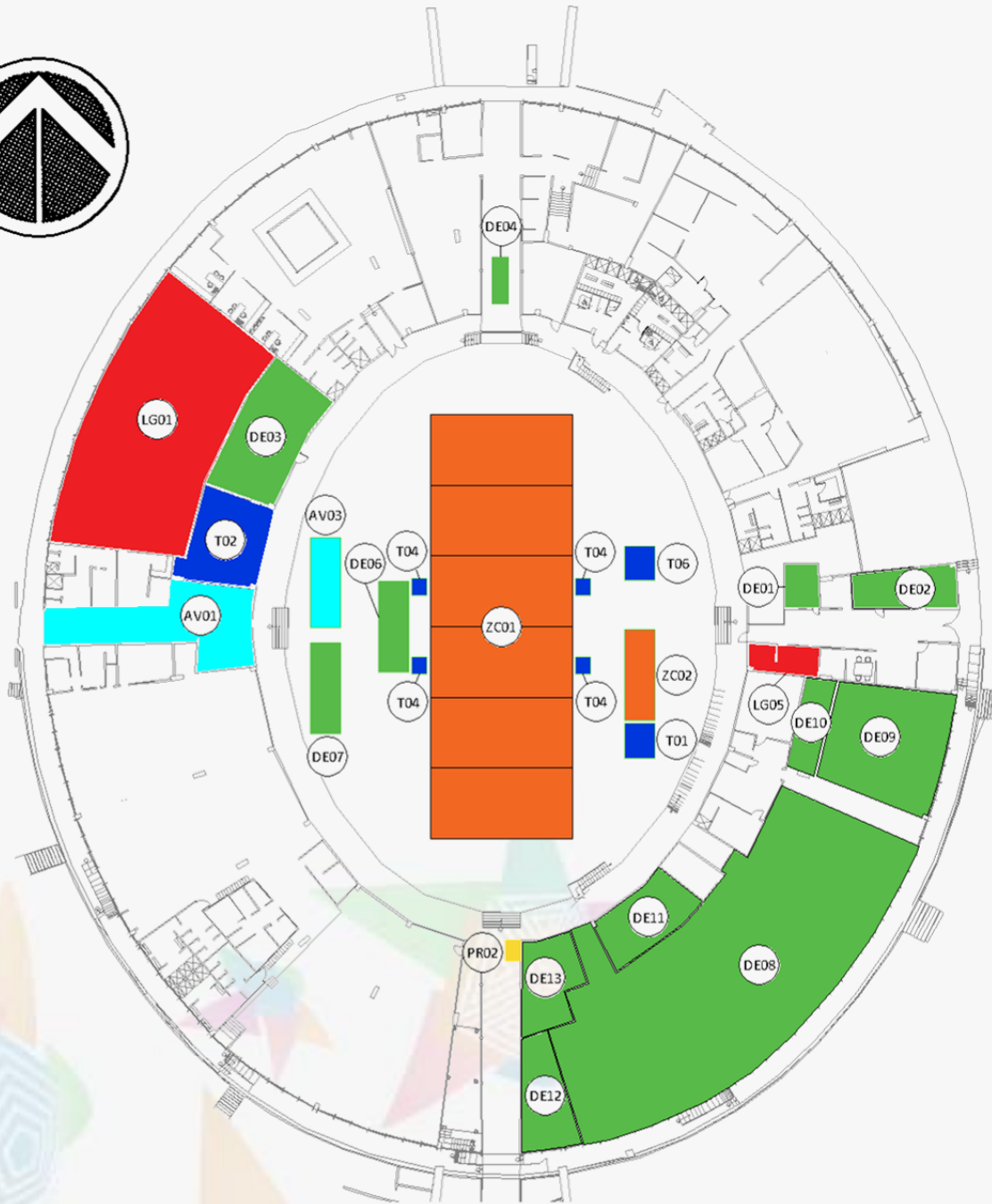
Figura 26 Layout tenis de mesa
