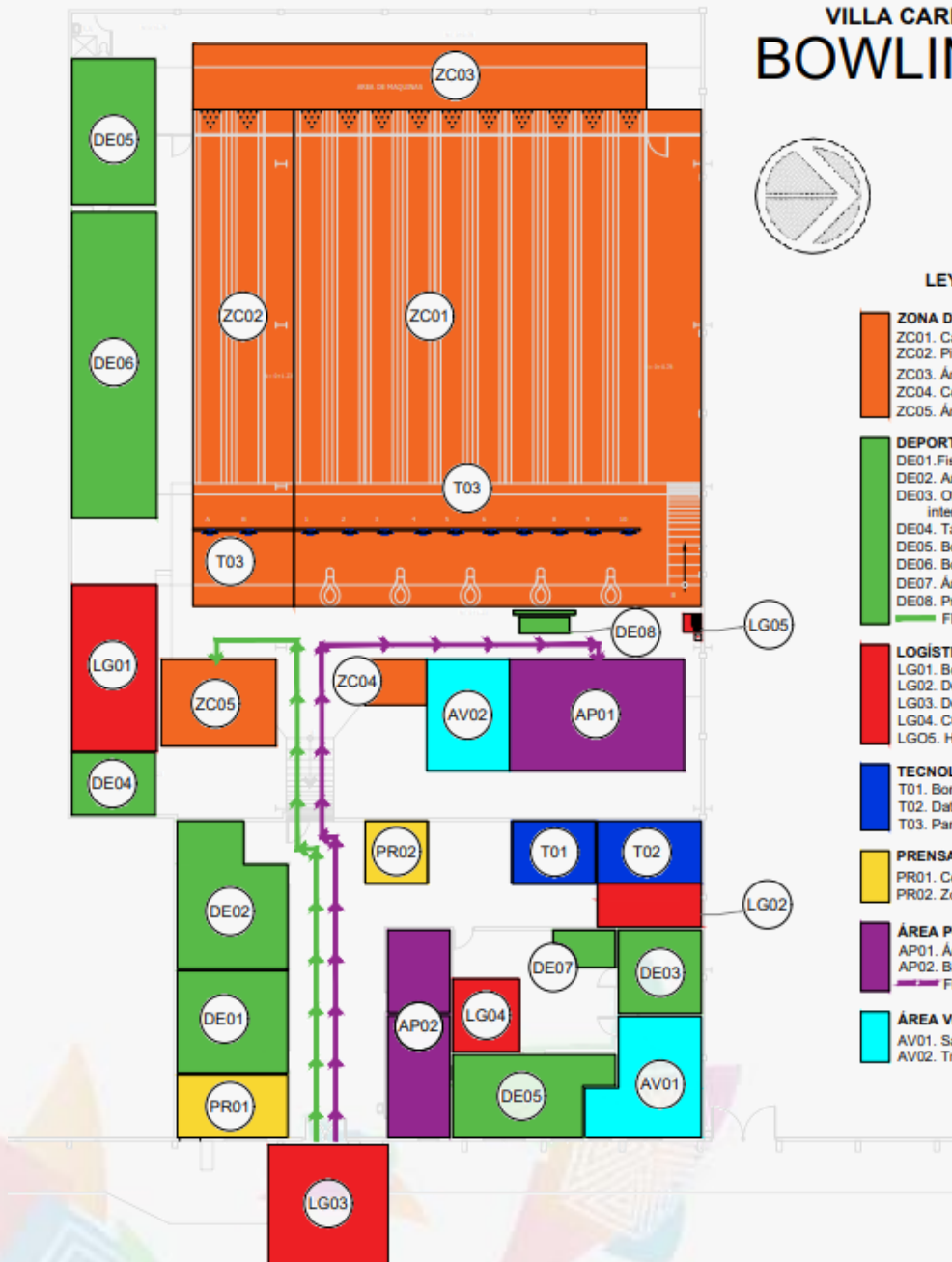
Figura 49 Layout boliche
