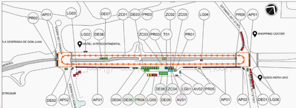
Figura 73 Patinaje de ruta vuelta al circuito
