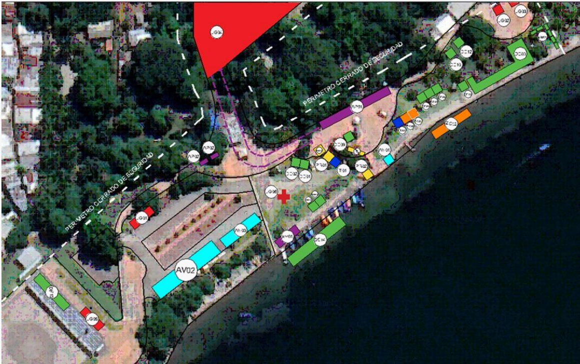
Figura 58 Layout aguas abiertas
