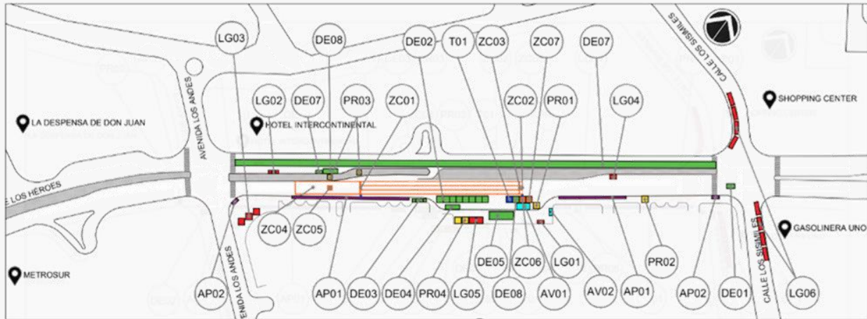
Figura 72 Layout patinaje de ruta 100 metros
