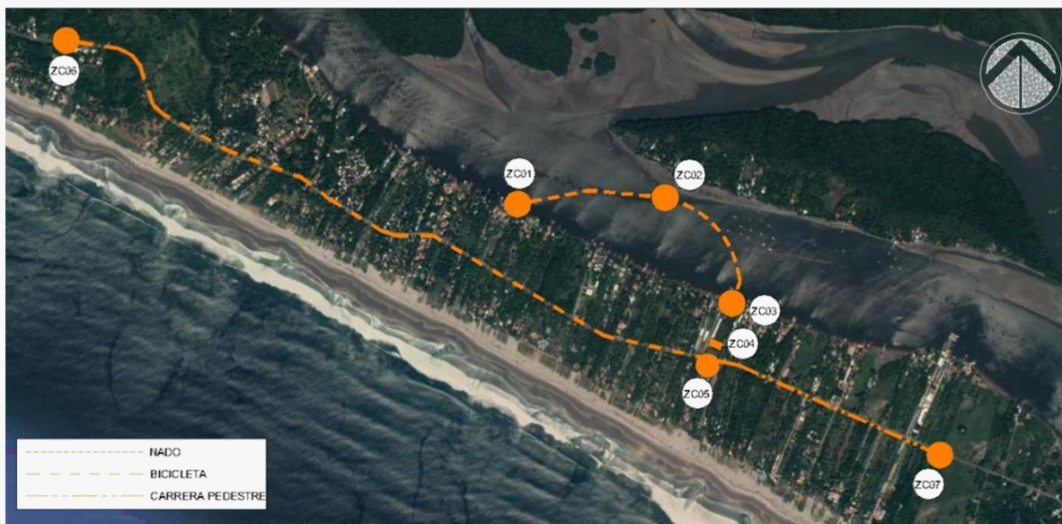
Figura 39 Layout triatlón
