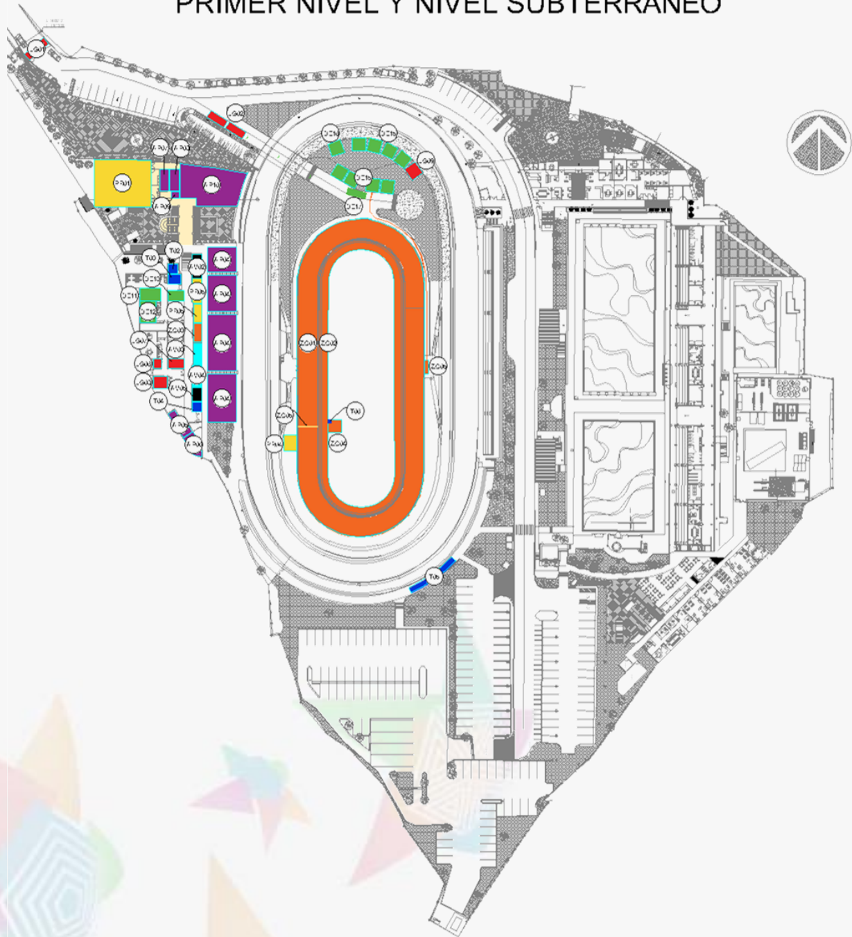
Figura 5 Layout patinaje velocidad
